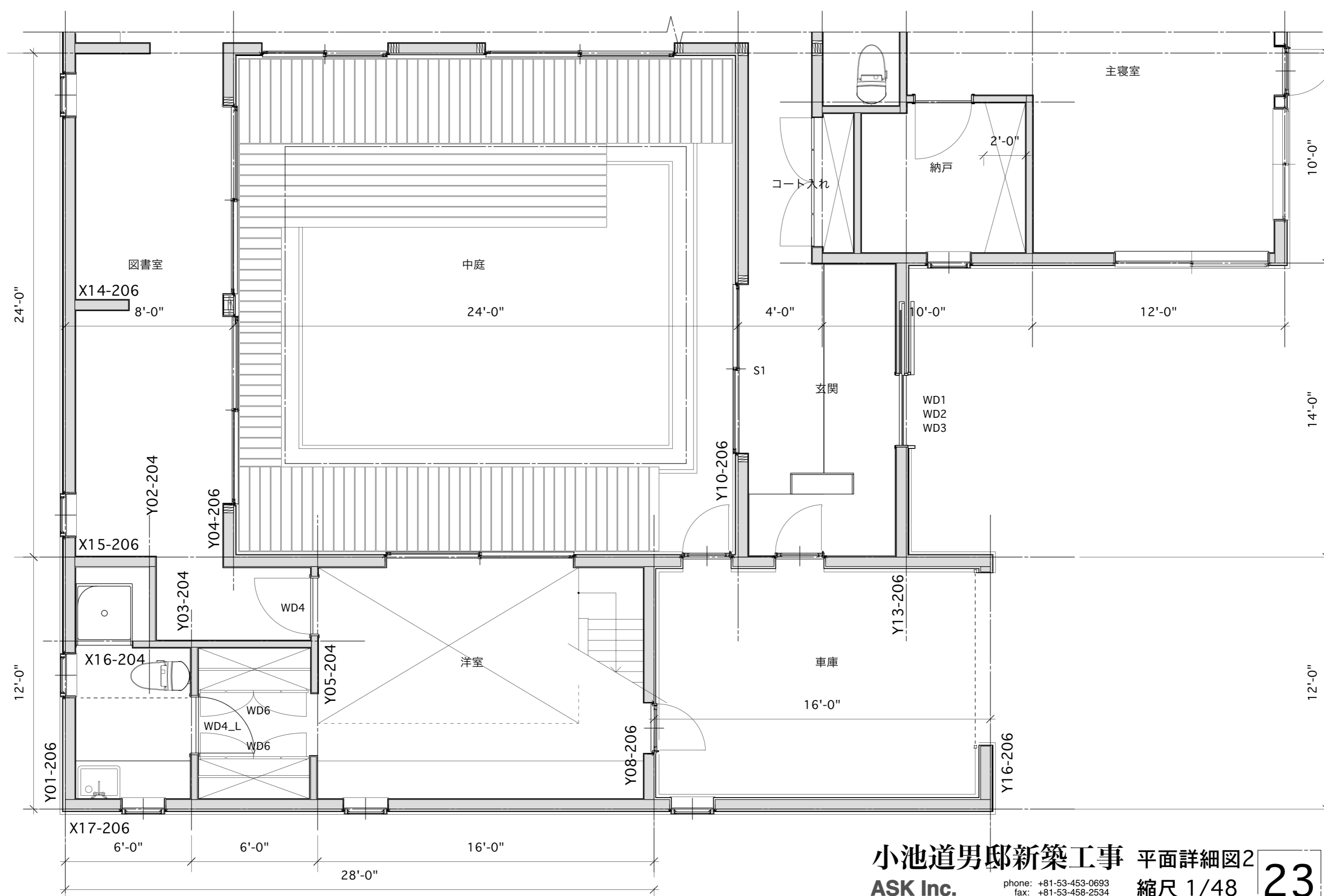
070203 バスルーム配置
