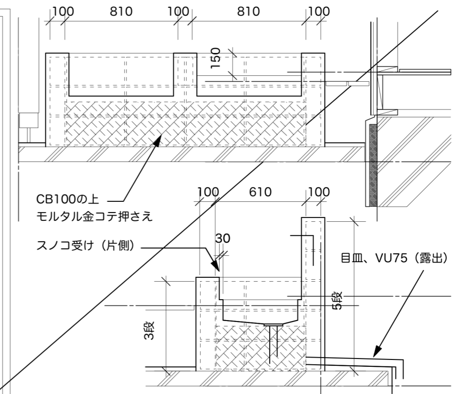
F 外流し部分詳細図 (別途) 1/25
