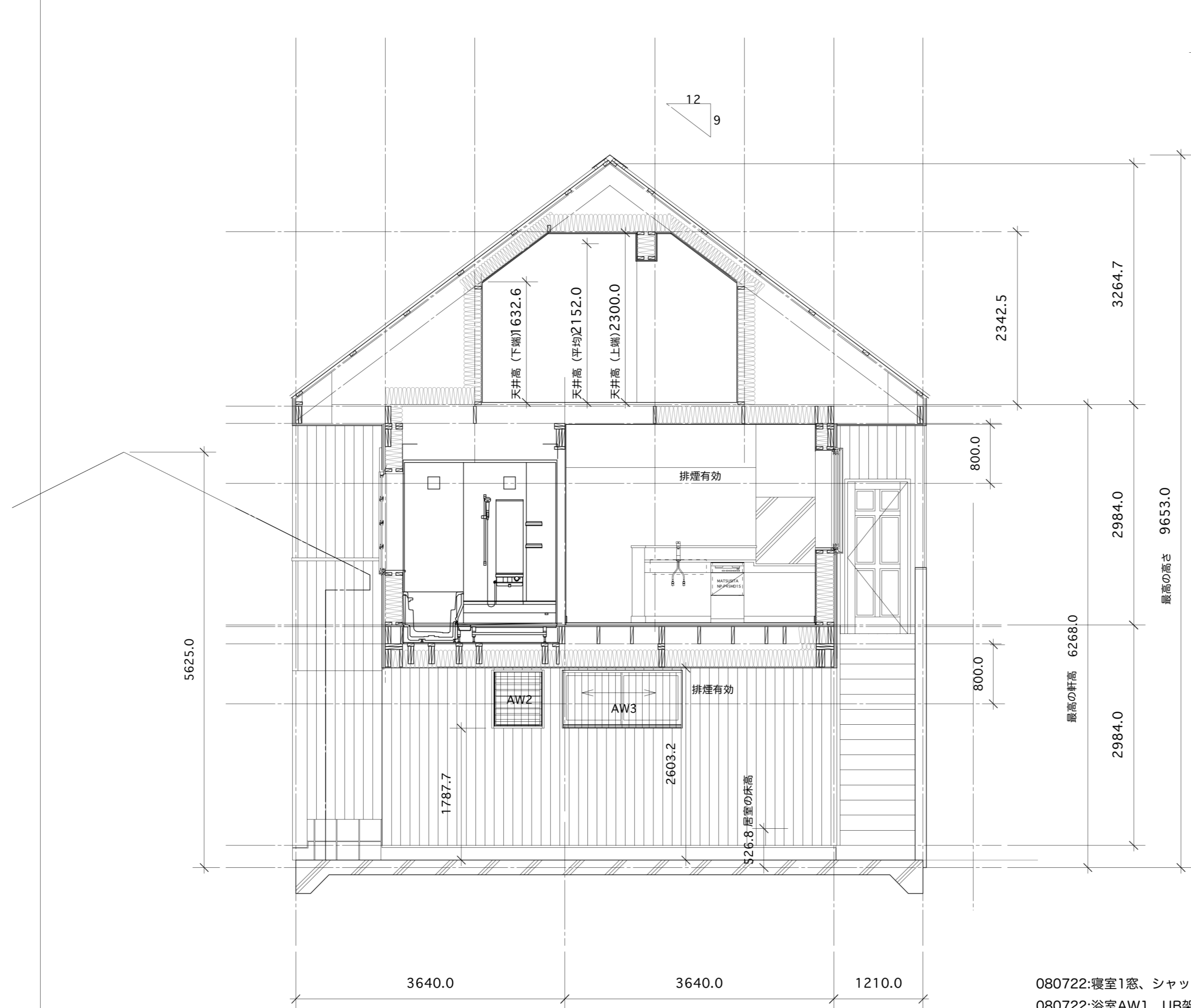
断面詳細図1 縮尺 1/50
