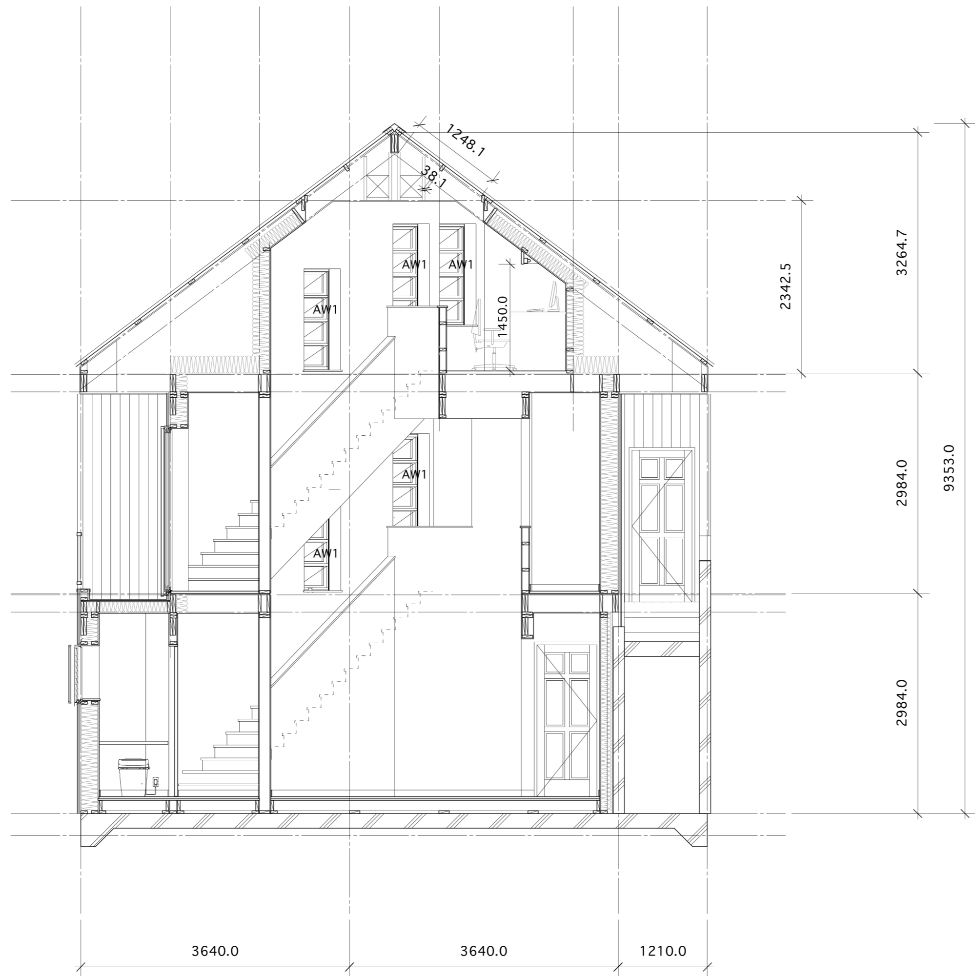
断面詳細図3 縮尺 1/50
