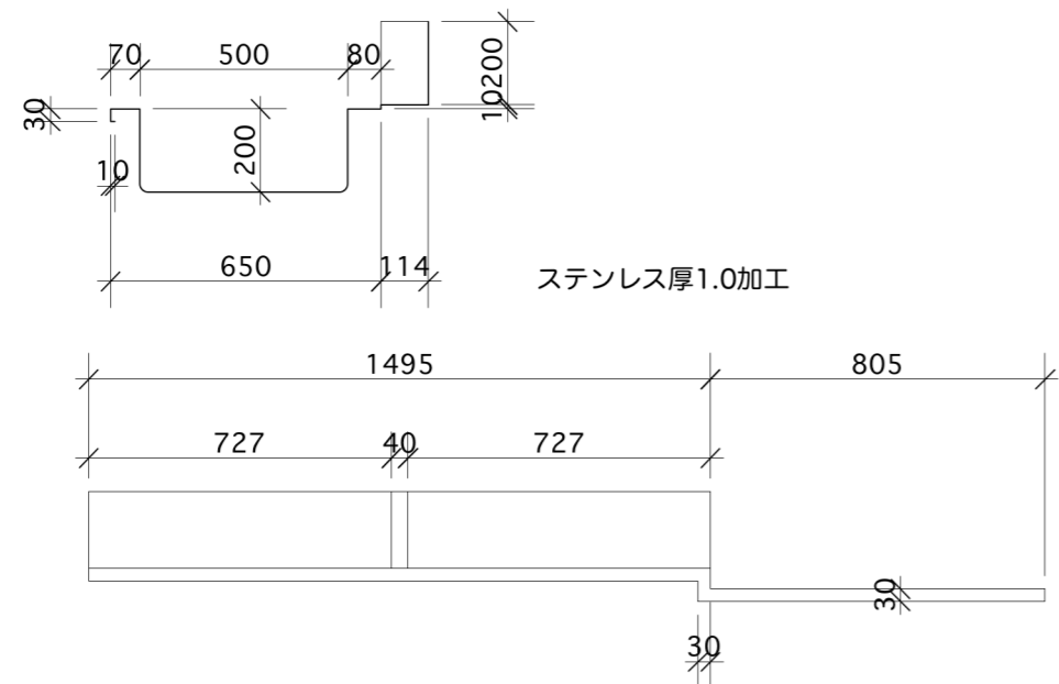
台所家具詳細図
