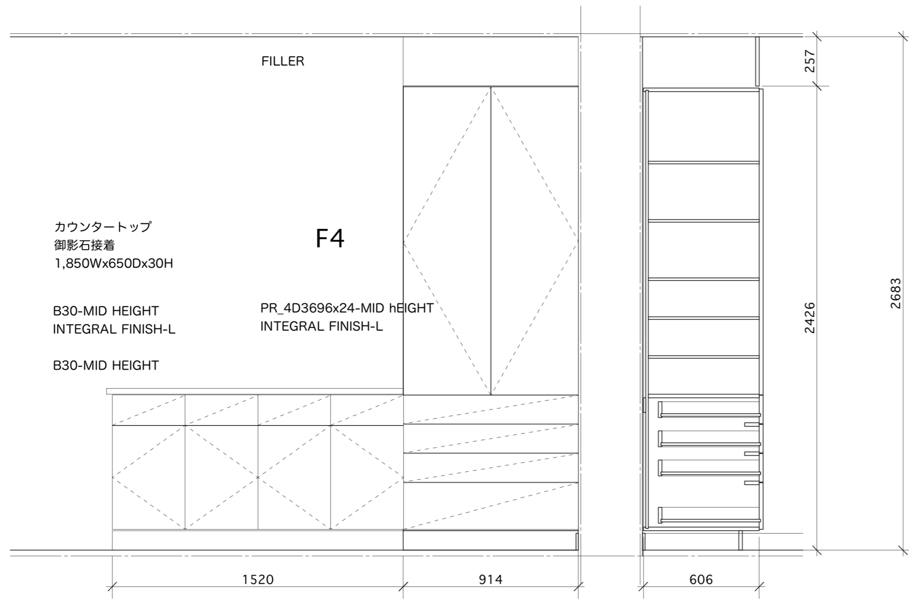
パントリー家具詳細図
