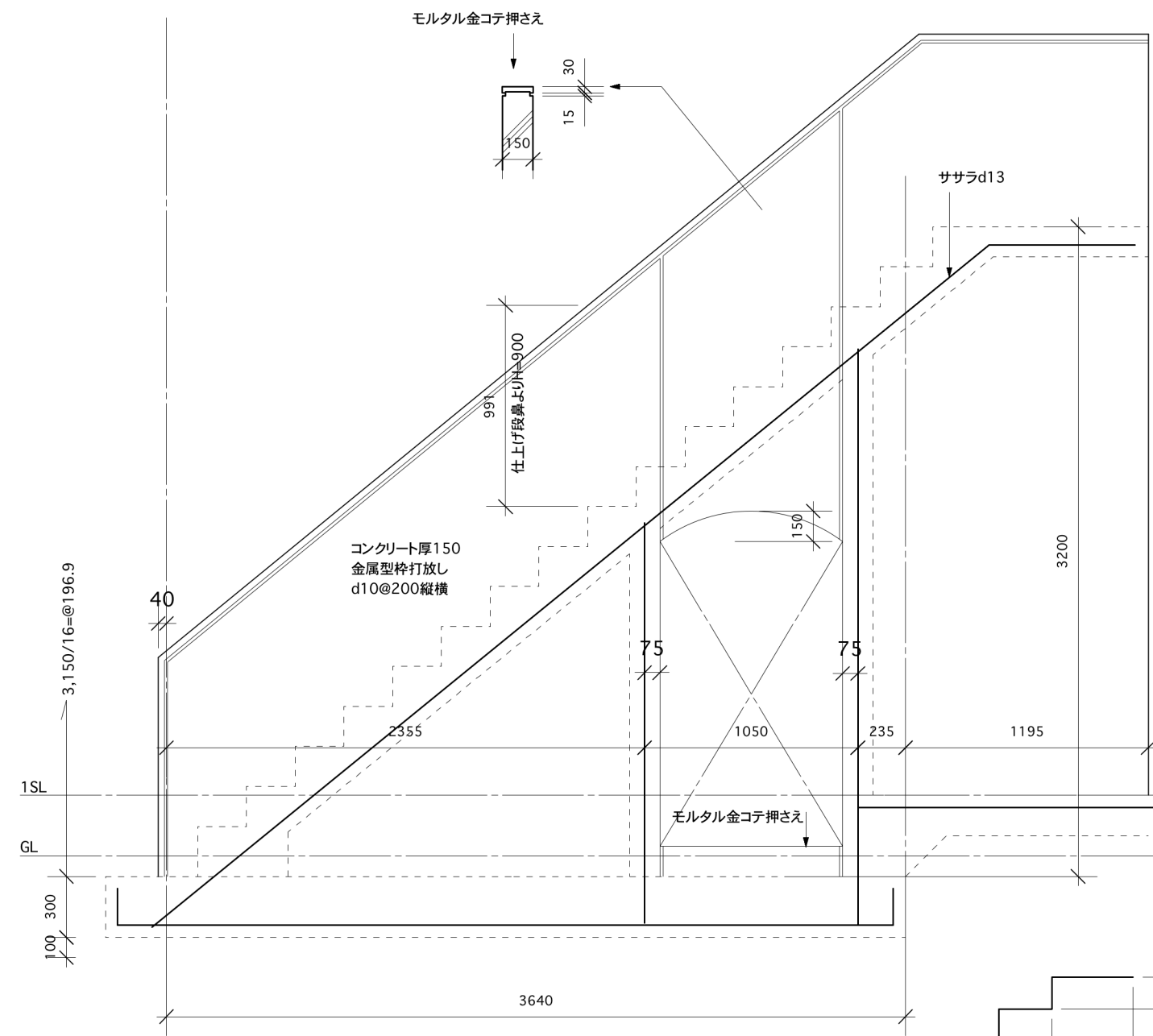
外部階段道路側部分詳細 1/30
