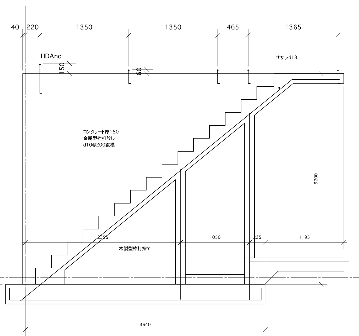
外部階段建屋側部分詳細 1/30
