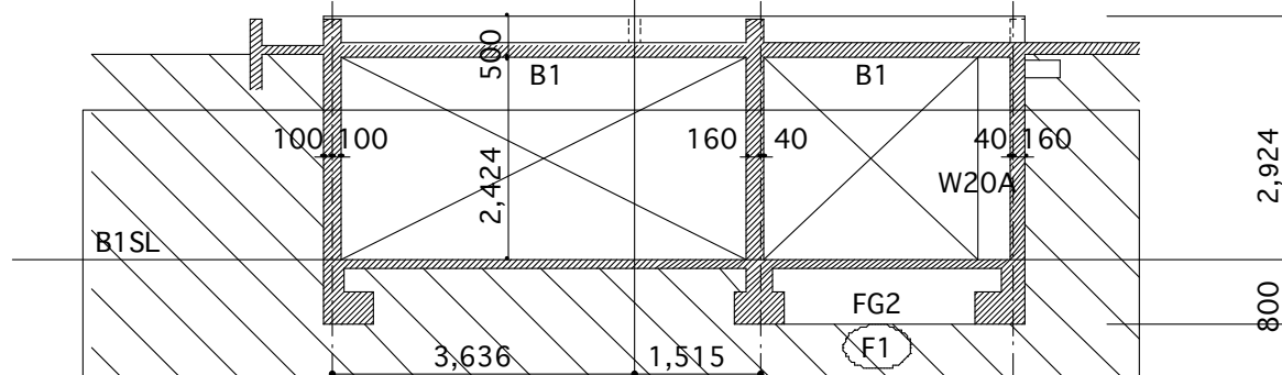
㌔ 通り軸組図 S=1/100
