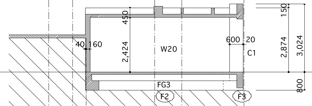
8 通り軸組図 S=1/100
