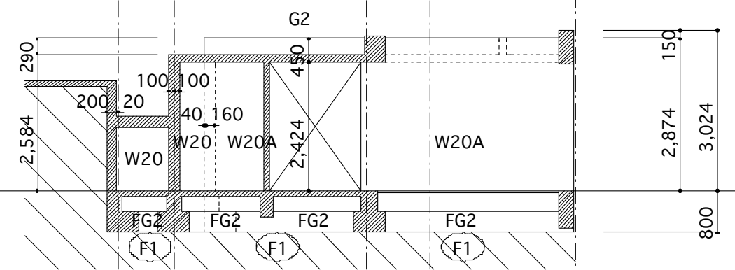
8 通り軸組図 S=1/100
