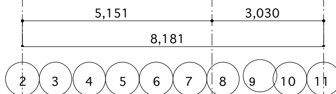
㌖ 通り軸組図 S=1/100
