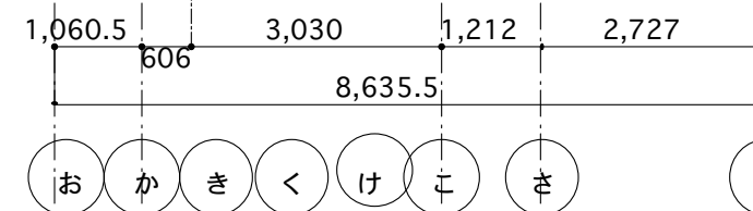
2 通り軸組図 S=1/100
