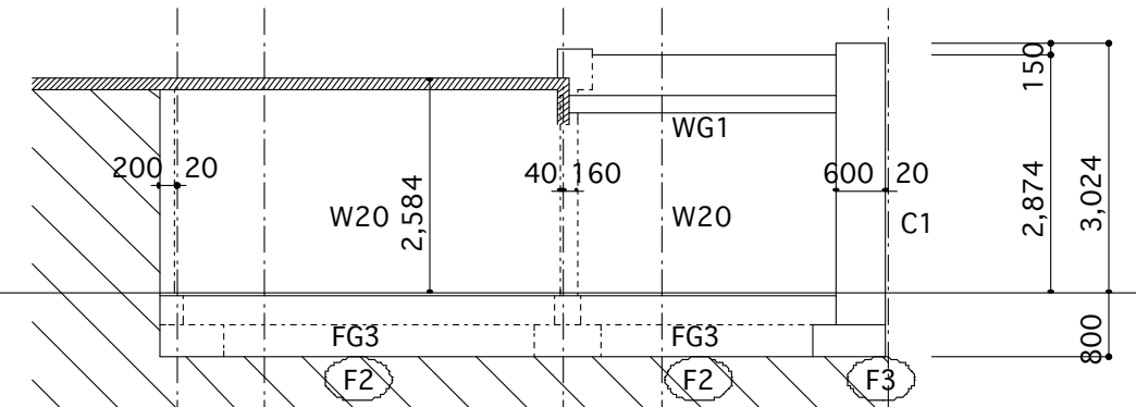
11 通り軸組図 S=1/100
