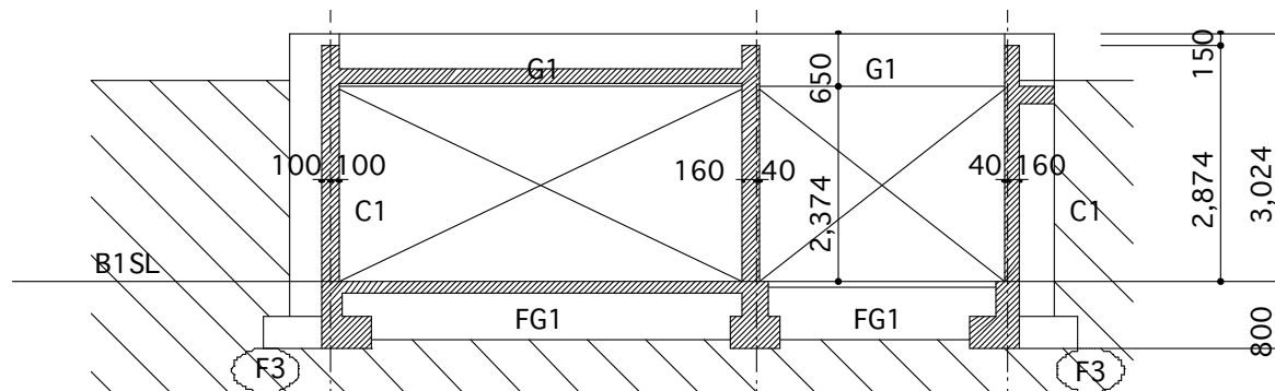
㌒ 通り軸組図 S=1/100
